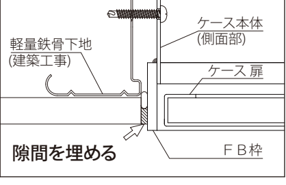
FBタイプ/ 標準納まり PAT.
