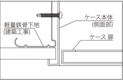
枠タイプ/ 標準納まり PAT.
