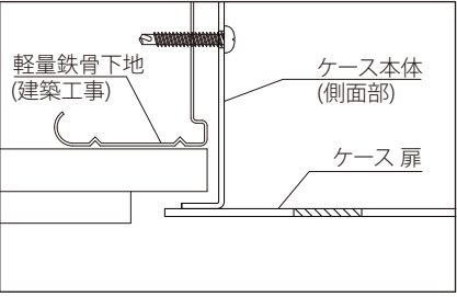
被せタイプ/ボード壁面面落ち納まり PAT.
