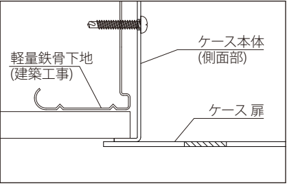
被せタイプ/ボード壁面標準納まり PAT.
