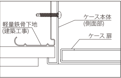
枠タイプ/ 面落ち納まり PAT.
