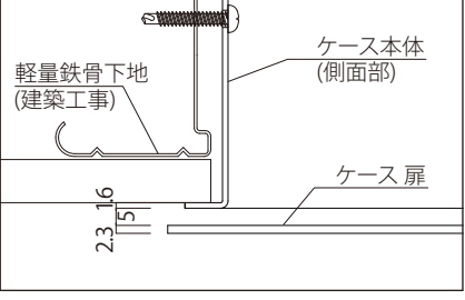
被せPUSHタイプ / 標準納まり PAT.
