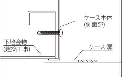
被せタイプ/パネル壁面標準納まり PAT.
