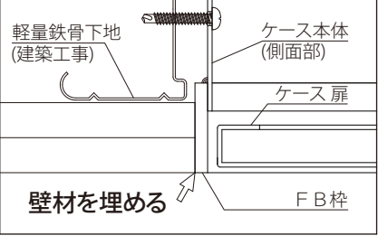
FBタイプ/ 同面納まり PAT. 消火器ケース 本体先行取付
