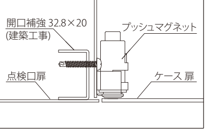
点検口扉に取付ける場合 PUSHタイプ/ 同面納まり PAT.
