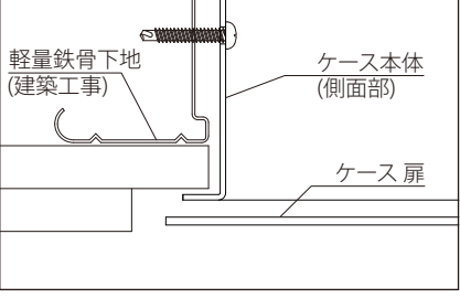
被せPUSHタイプ/ 面落ち納まり PAT.
