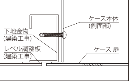
被せタイプ/パネル壁面同面納まり PAT.
