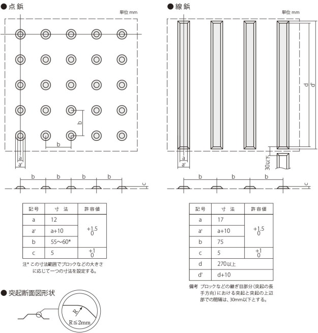
JIS規格製品の形状・寸法及びその配列
